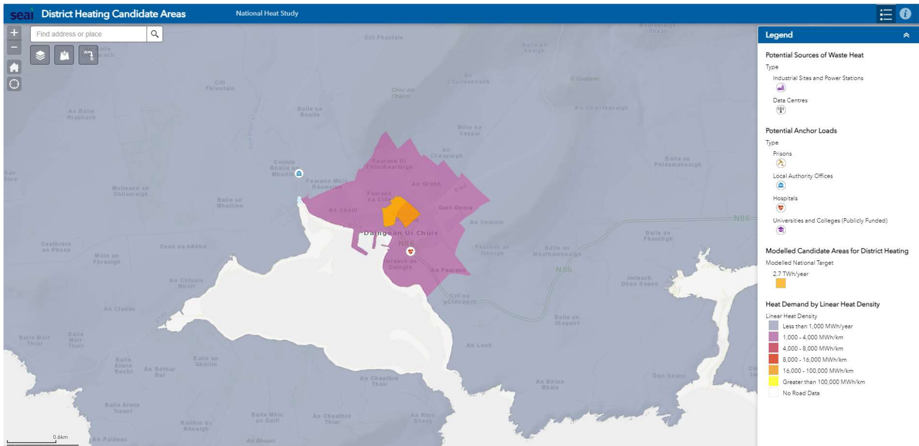
Fíor 6-3 Léarscáil SEAI (Údarás Fuinnimh Inmharthana na hÉireann) ar Limistéir Iarrthóireachta um Théamh Ceantair ina sainithnítear Daingean Uí Chúis mar limistéar féideartha iarrthóireachta 20
