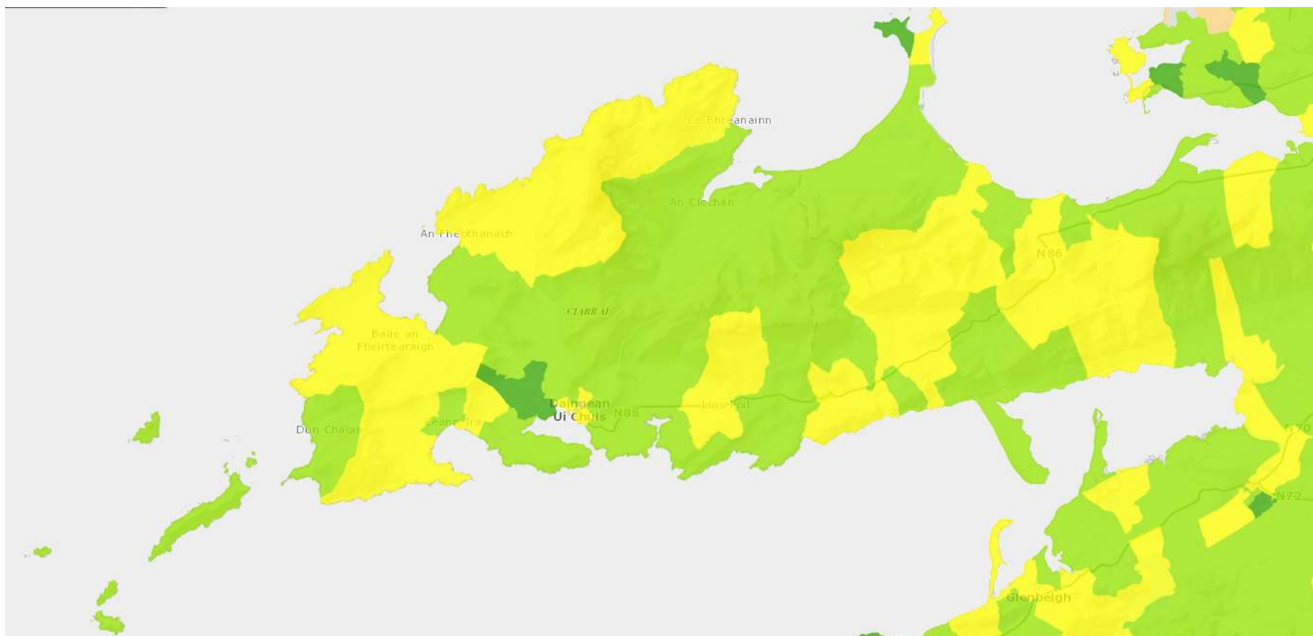
Fíor 6-2 Léarscáil SEAI (Údarás Fuinnimh Inmharthana na hÉireann) ina dtaispeántar Rátálacha Fuinnimh Foirgnimh (BER) ar fud na leithinse - BER C (glas) agus BER D (bui) 19
