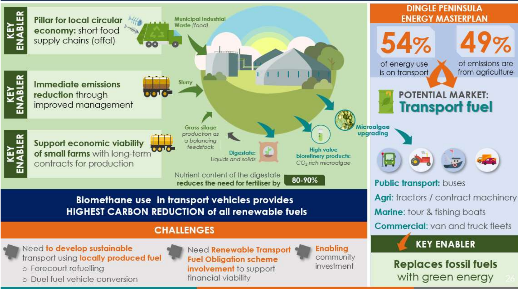
Fíor 6-4 Acmhainneacht an bhithmheatáin in DZ Dhaingean Uí Chúis/Corca Dhuibhne mar atá sainaitheanta ag an bpobal
