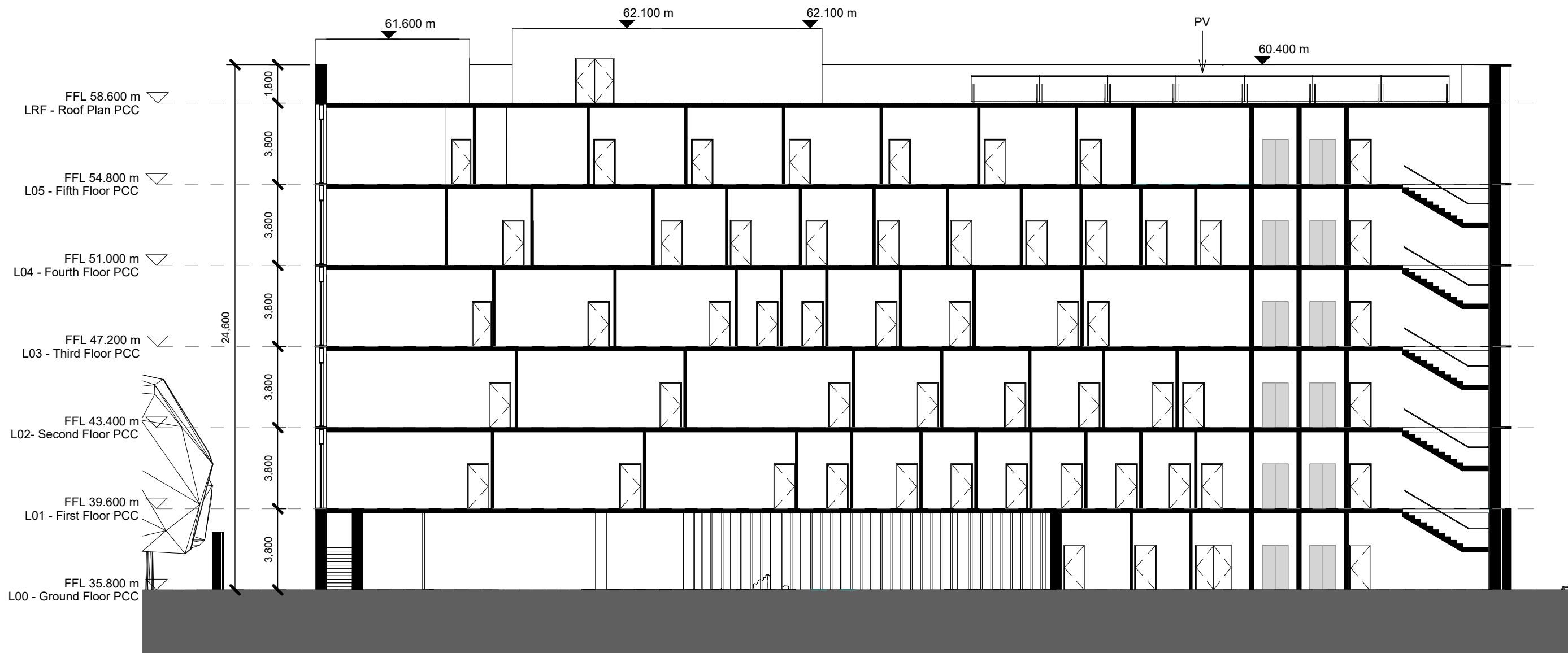
Section A PCC 1 : 200
