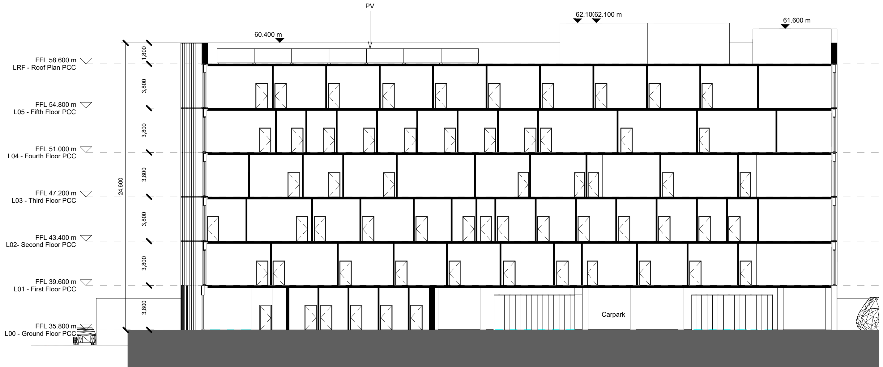
Section B PCC 1 : 200
